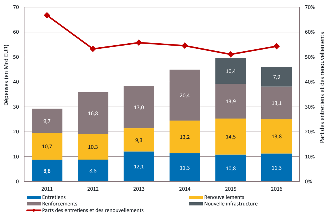
Graphique 10: Évolution des dépenses d'infrastructure et proportion des dépenses d'entretien et de renouvellement sur la période 2011-2016
