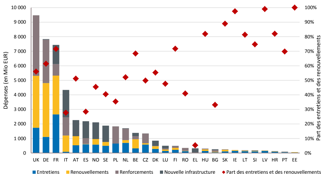
Graphique 11: dépenses d'infrastructure et part des dépenses d'entretien et de renouvellement par pays, 2016
